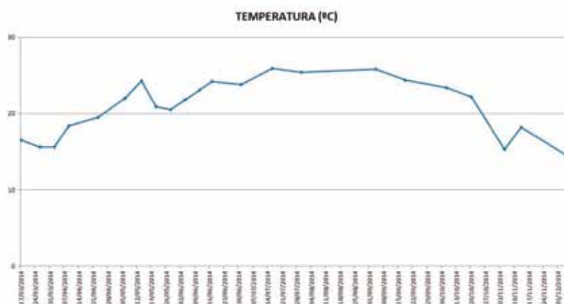
FIGURA 5. Evolución de la temperatura del agua durante el periodo de estudio.
